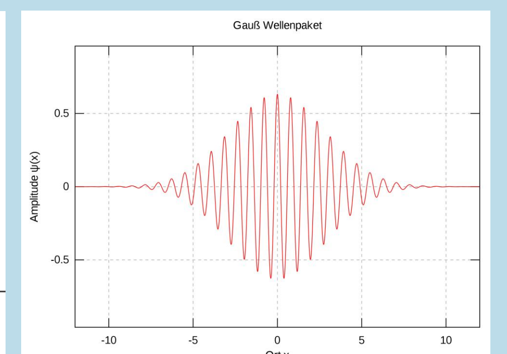
Abb. 3: Gauß'sches Wellenpaket
