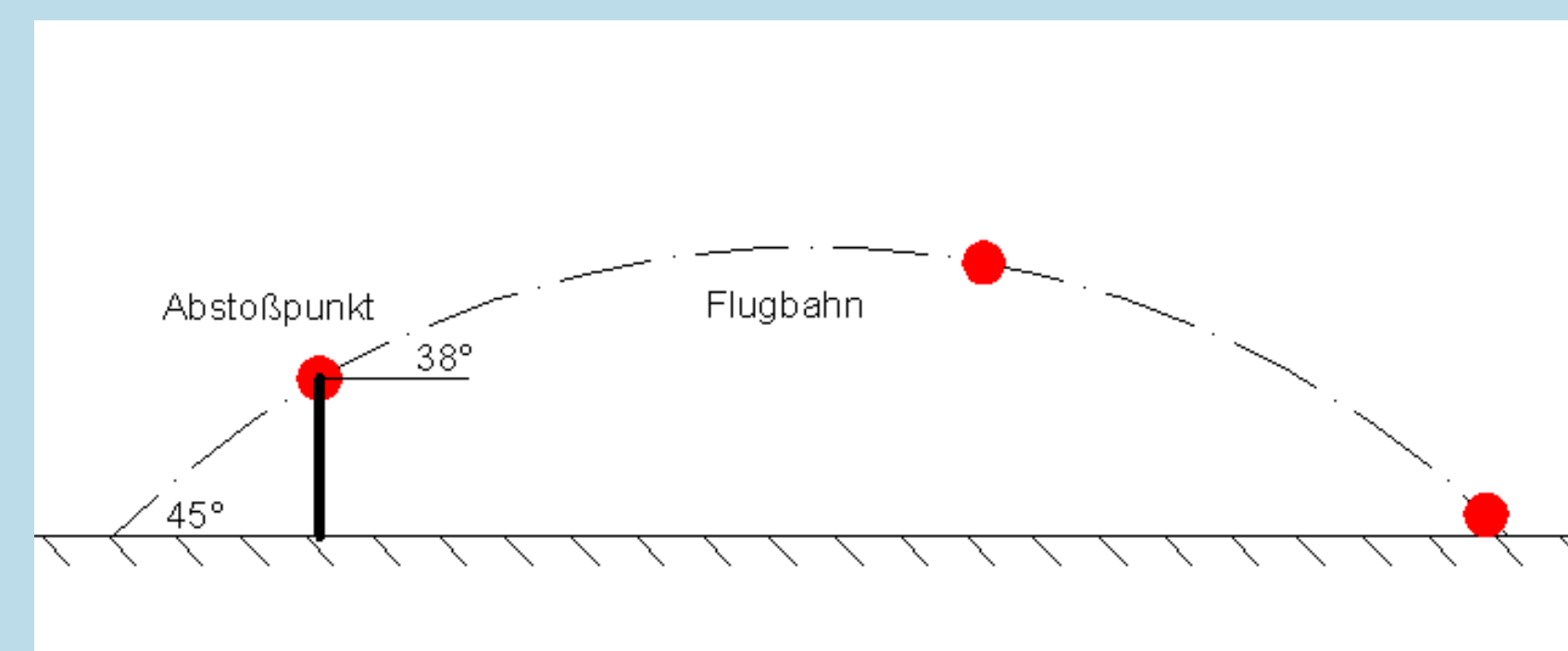
Abb. 2: Ballwurf
