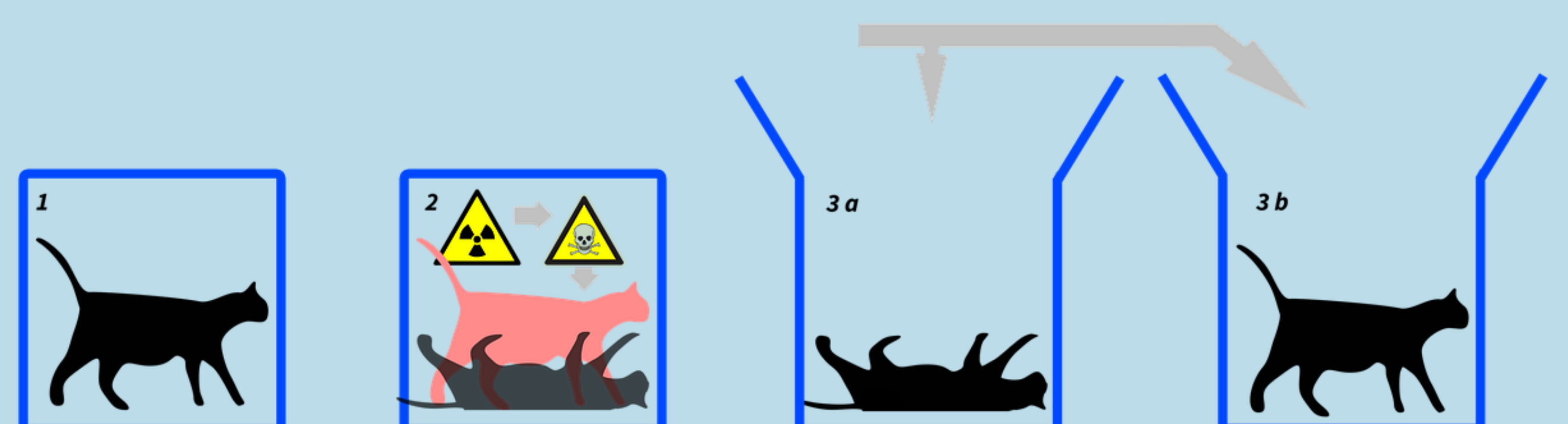
Abb. 5: Schrödingers Katze
